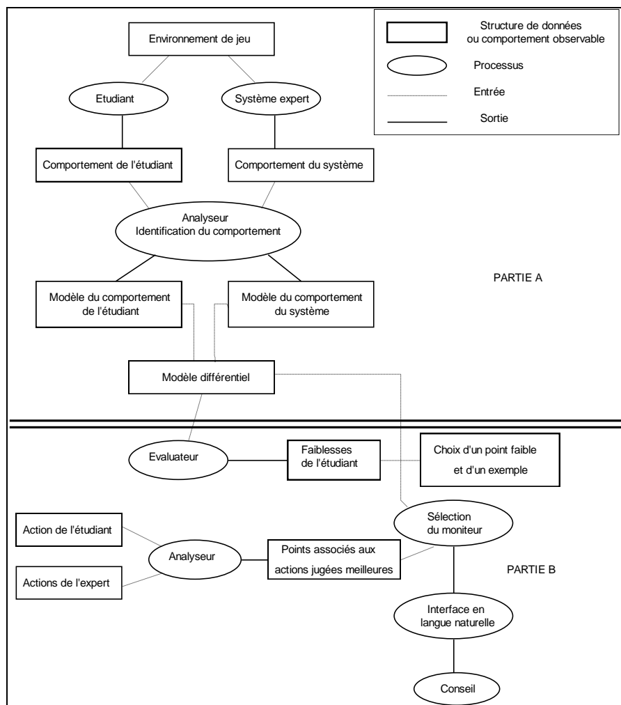
Figure 3.3. Diagramme des processus de modélisation et d'intervention dans WEST (Burton et Brown, 1982)
